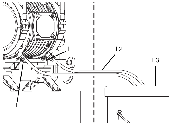
ŞEKİL 6: Sıvı Sızıntı Hatlarının Tipik Montajı (Normal Konumlar)
