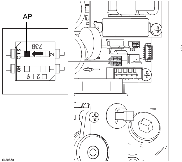
ŞEKİL 12: Otomatik Doldurmanın Devre Dışı Bırakılması
