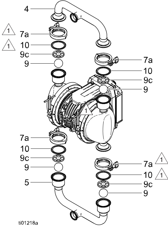
ŞEKİL 16: Çek Valfler (HS Küresel Pompalar)
