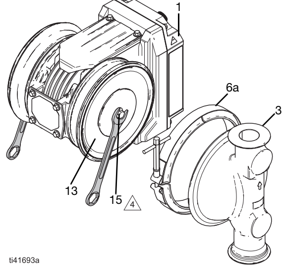
ŞEKİL 21: Standart Diyaframların Sıkılması
