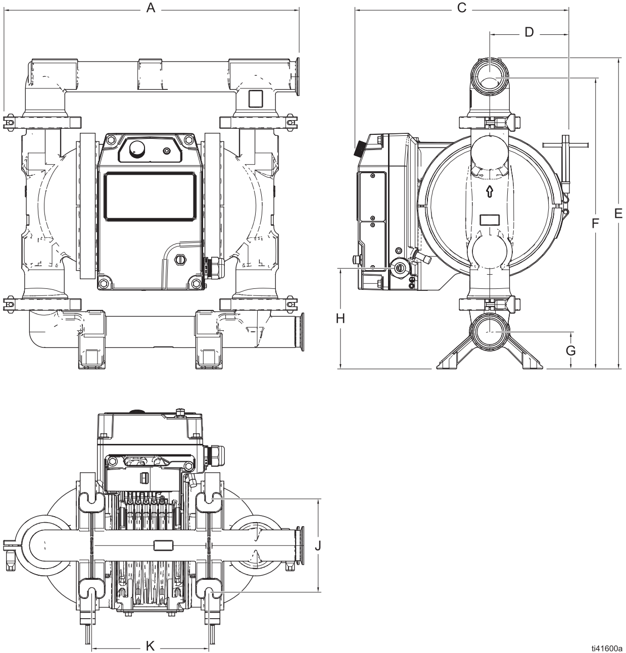
ŞEKİL 27: h80 (QHD) Model Boyutları (FG modeli gösteriliyor)
