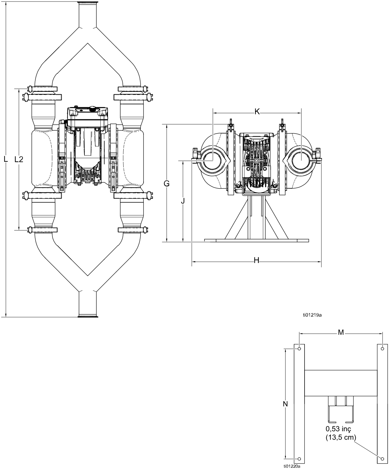
ŞEKİL 31. h120 (QHF) Yatay Kanatlı Model Boyutları (SSE modeli gösterilmiştir)
