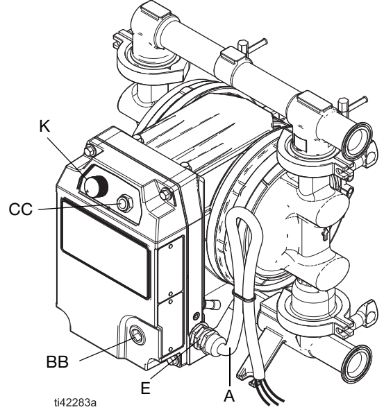
ŞEKİL 2: Patlayıcı Ortamlar veya Tehlikeli (Sınıflandırılmış) Konumlarda Kullanılan Model (h30 (QHC) modeli gösteriliyor)
