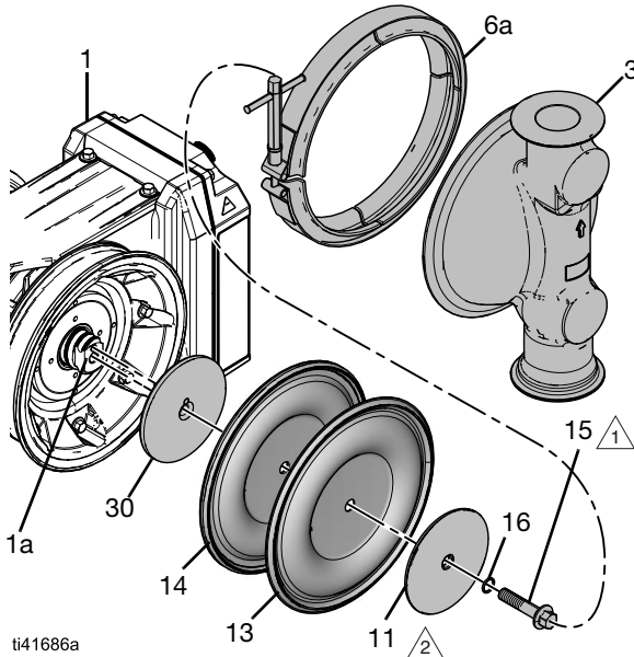
ŞEKİL 20: Standart Diyaframların Yeniden Monte Edilmesi (Hijyenik Model Gösteriliyor)
