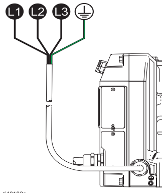
ŞEKİL 10: 3 Fazlı Modellerin Bağlanması
