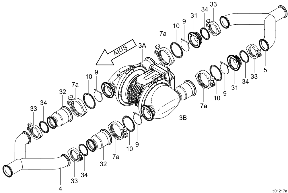
ŞEKİL 18: Çek Valfler (Yatay Kapaklı Pompa)
