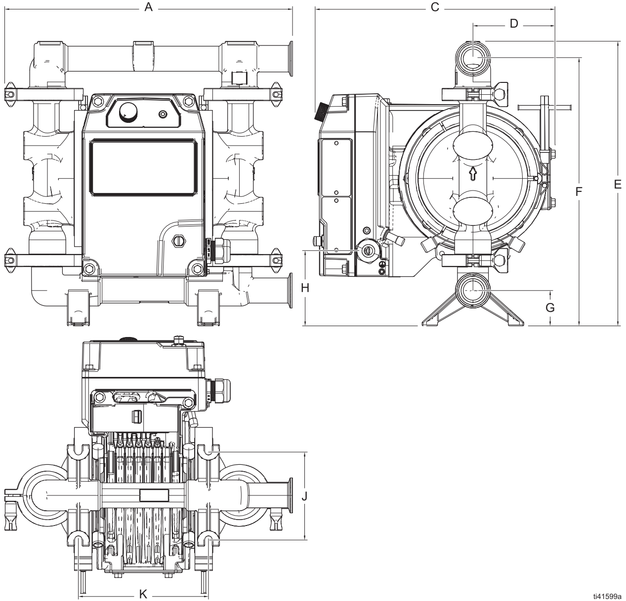
ŞEKİL 25: h30 (QHC) Hijyenik Model Boyutları (FG modeli gösteriliyor)
