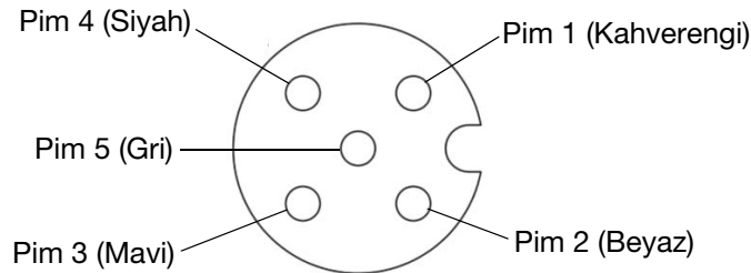
ŞEKİL 11: Normal Konumlarda Kullanılan Modeller İçin 5 pimli M12 Konektörü
