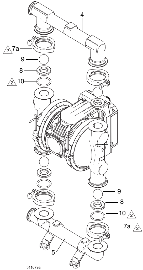
ŞEKİL 15: Çek Valfler (FG Küresel Pompalar)
