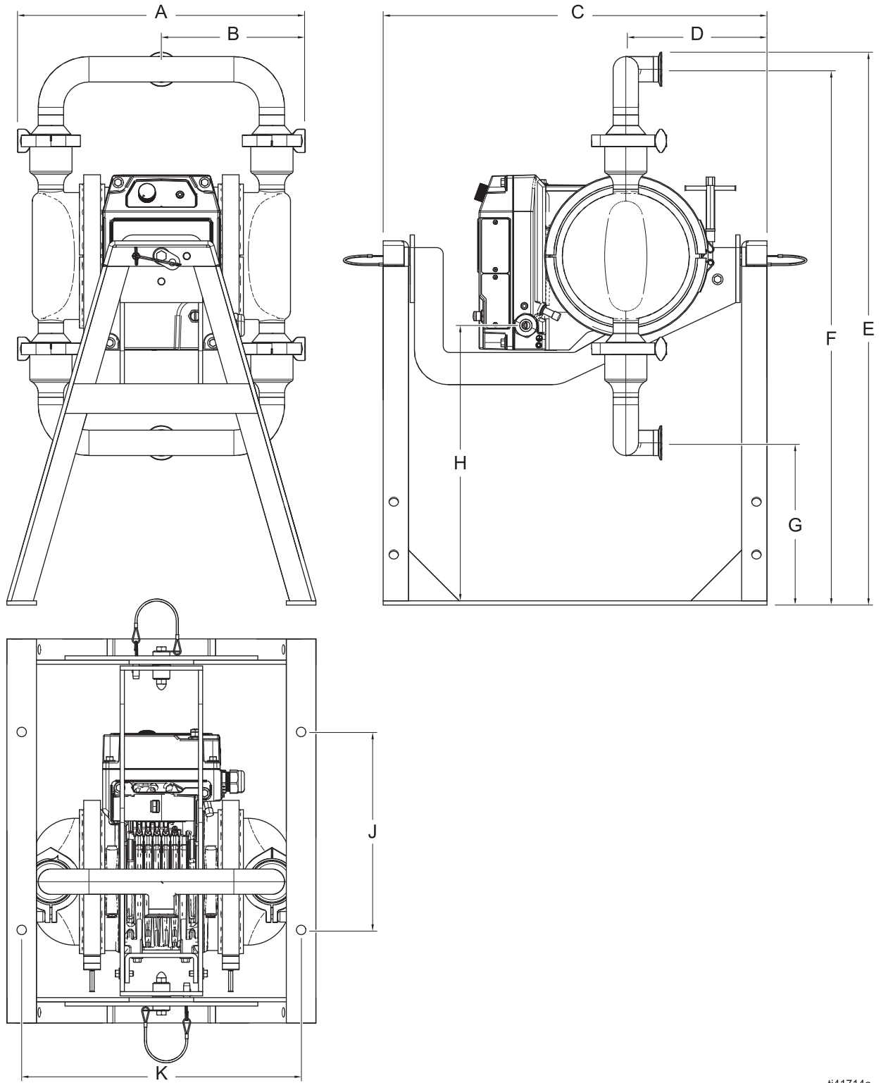
ŞEKİL 28: h80 (QHD) Model Boyutları (HS modeli gösteriliyor)
