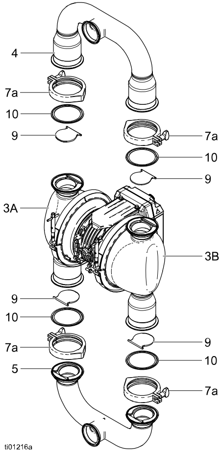
ŞEKİL 17: Çek Valfler (Dikey Kapaklı Pompa)
