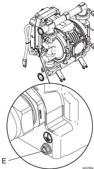
ŞEKİL 7: Ekipman Toprak Bağlantı Elemanı
