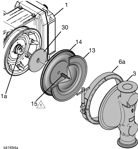
ŞEKİL 23: Enjeksiyonlu Kalıp Diyaframlarının Yeniden Monte Edilmesi
