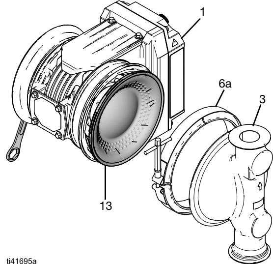
ŞEKİL 24: Enjeksiyonlu Kalıp Diyaframların Sıkılması
