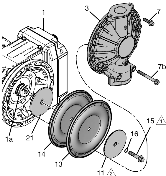
ABB. 20: Standard-Membranen zusammenbauen
