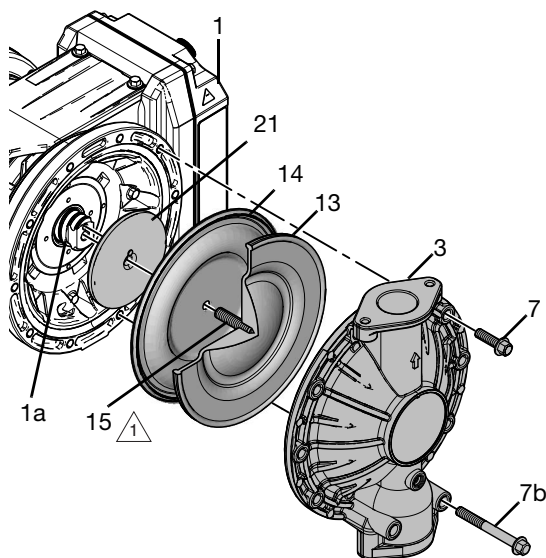
ABB. 23: Einbau – umgossene Membranen
