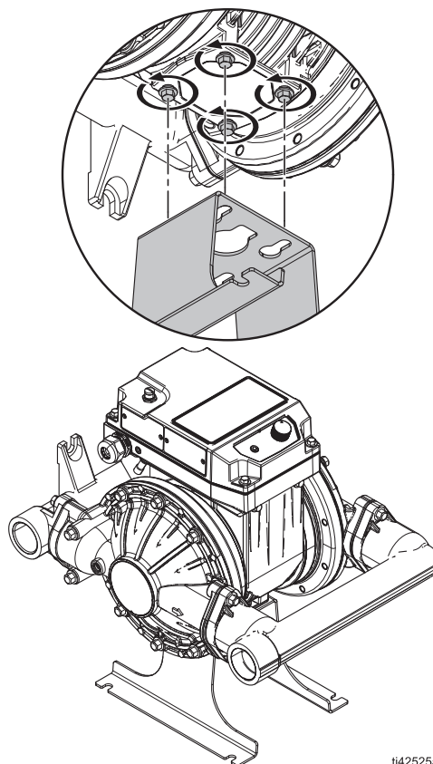
ABB. 16: Ständer der Wartungshalterung
