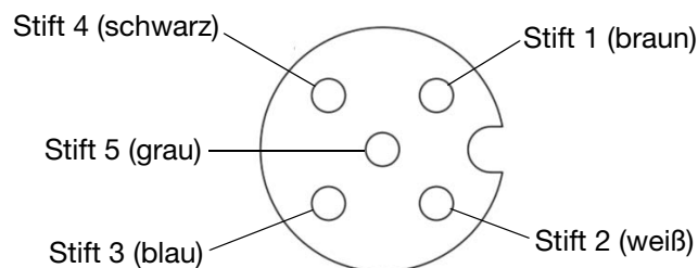
ABB. 14: M12, 5-poliger Stecker für Modelle an gewöhnlichen Standorten Ausrichtung: in Richtung des Steckers am Pumpenkörper.
