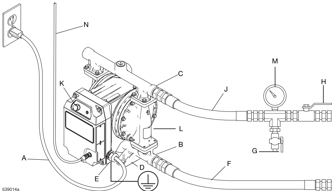
ABB. 3: Typische Installation für Modelle an gewöhnlichen Standorten (Kabel- und Steckeranschluss) (Modell i30 (QTC) abgebildet)
