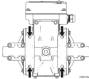
ABB. 7: Montagebohrungen
