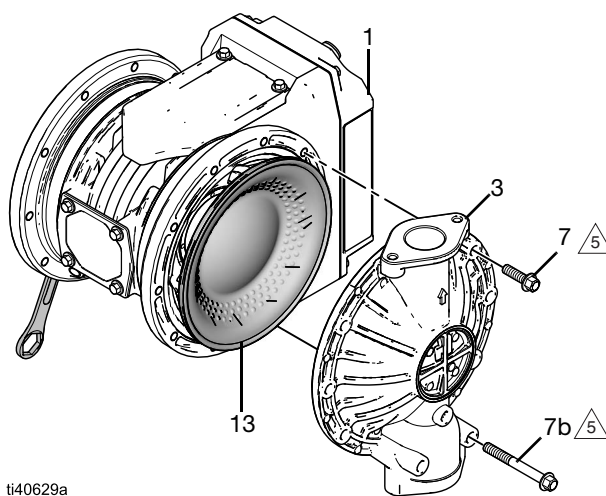
ABB. 24: Einbau – umgossene Membranen
