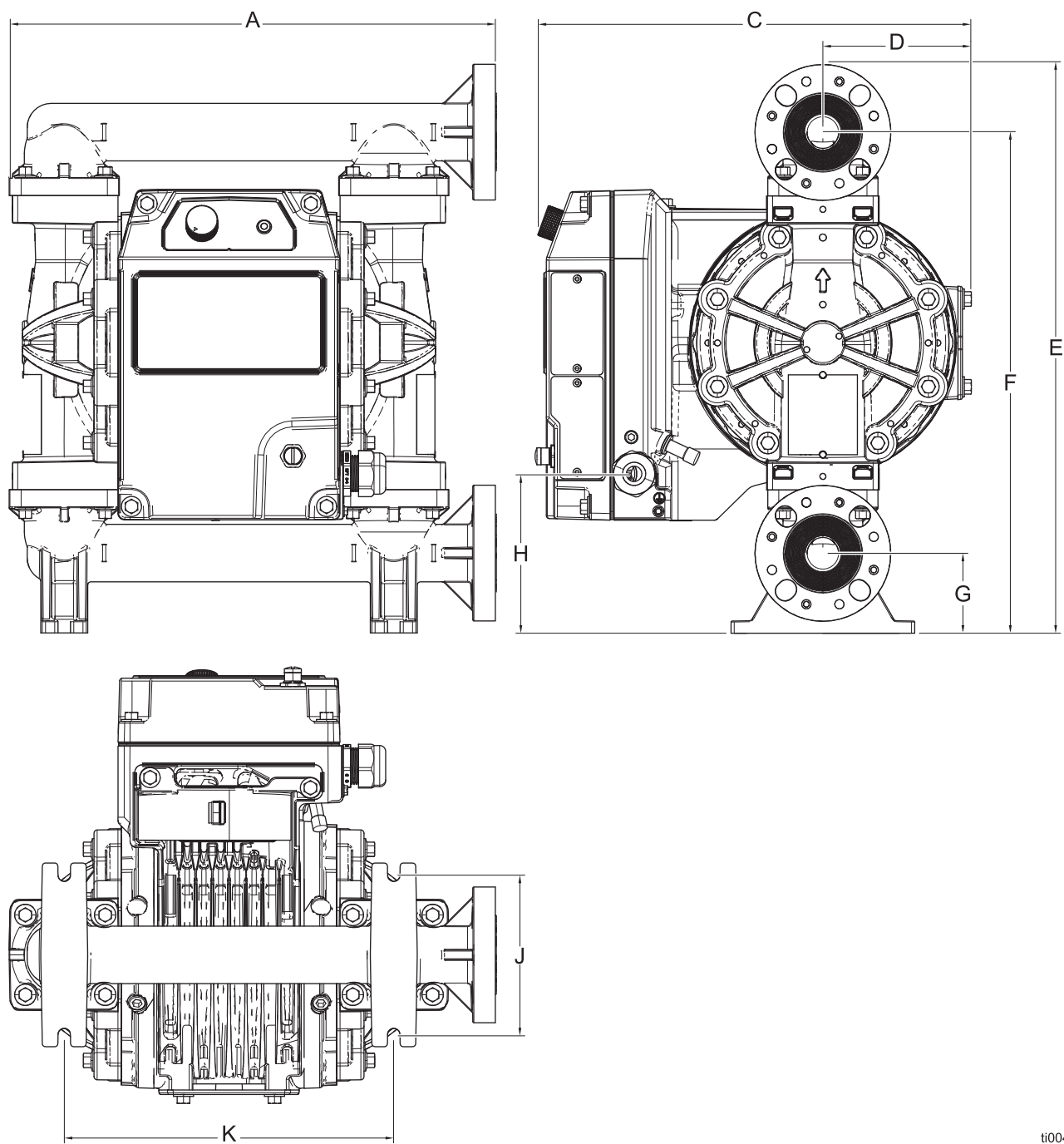
ABB. 26: Abmessungsdiagramm für i30 (QTC) mit materialberührtem Abschnitt aus Kunststoff, Endflansch
