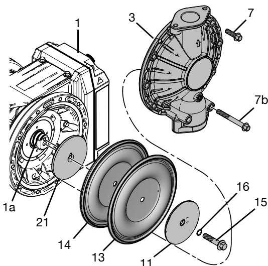
ABB. 19: Standard-Membranen
