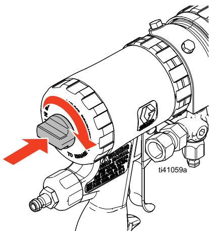
Le pistolet Fusion AP est illustré.
