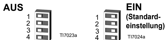
ABB. 46. Einstellungen des DIP-Schalters (SW2)
