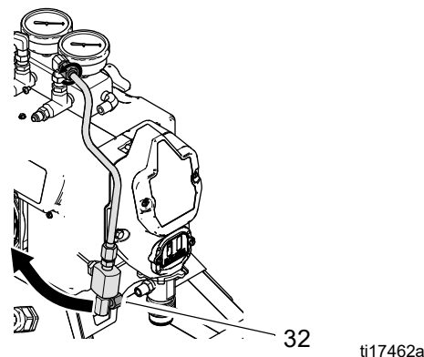
ABB. 51: Materialauslassleitung
