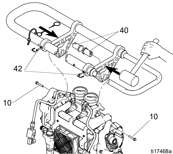
ABB. 58: Entfernen des Fahrgestellgriffs
