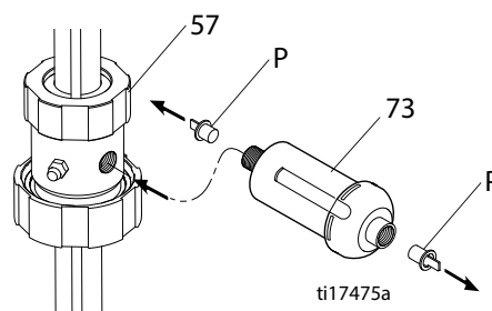
Рис. 6: Установка влагопоглотителя
