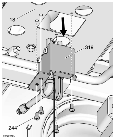
Изглед на ThermoLazer 300TC/ProMelt
