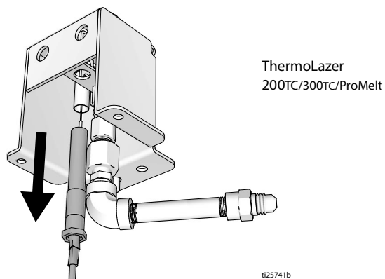
Изглед на ThermoLazer 300TC/ProMelt
