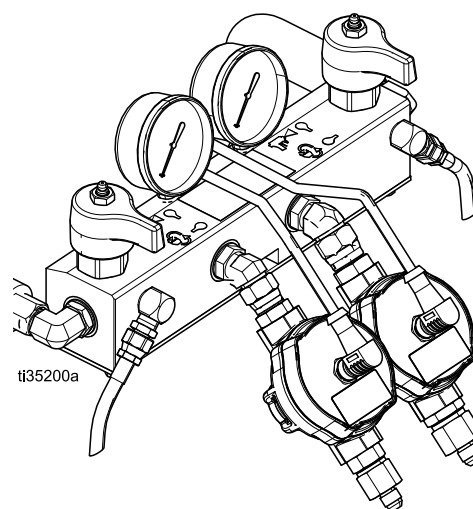
OBR. 7: Průtokoměr
