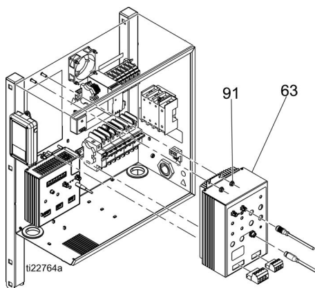
OBR. 20: Vyměňte modul MCM
