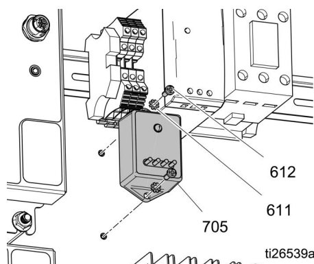
OBR. 19: Svodič přepětí
