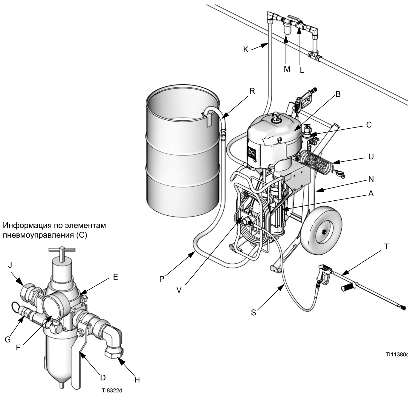
Рис. 1: Типовая установка оборудования (показан аппарат для монтажа на тележке)
