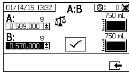
중량에서의 시스템 비율 모드
