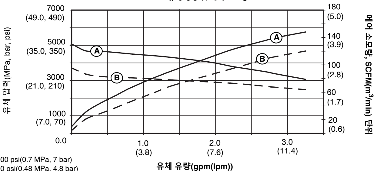
XM50 유체 성능 및 에어 소모량
