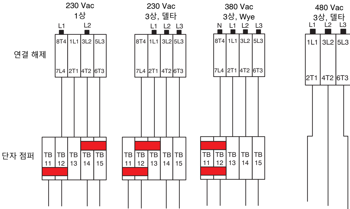
그림 7: XM 배선도
