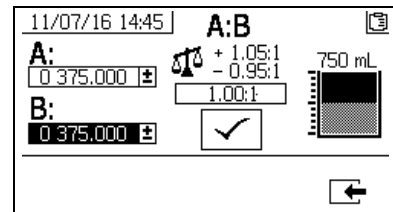
부피의 시스템 비율 모드 - 중량으로 테스트
