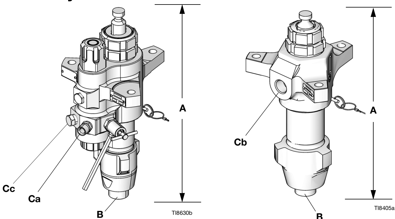
Distribučné jednotky so vstavanými filtrami
