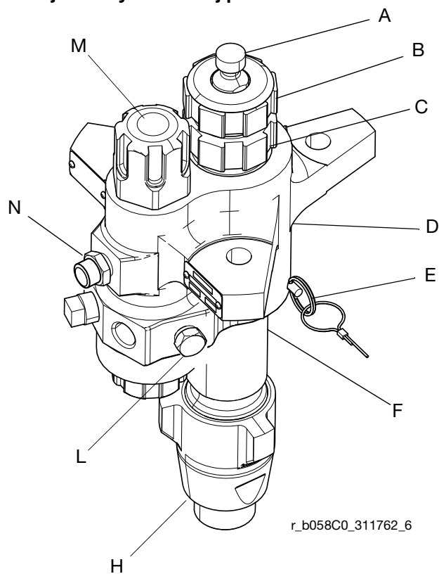
Distribučné jednotky Xtreme striekej pištole XP a distribučné jednotky striekej pištole e-Xtreme
