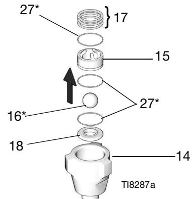
图 1: 拆除 Xtreme 下缸体
