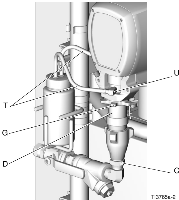
Rys. 1 Odłączenie pompy A
