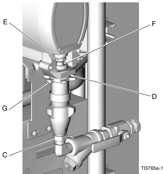
Rys. 2 Odłączenie pompy B
