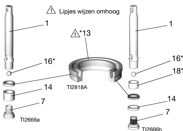
Typische configuratie
