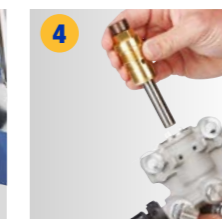
Neue Patrone installieren und Pumpe einsetzen
