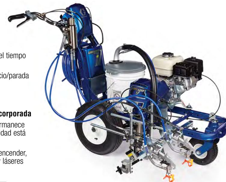
Se muestra el LineLazer V 5900 HP Automatic
