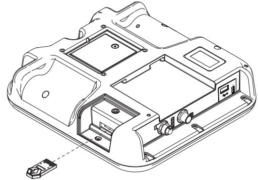
FIG. 8: Insert Token
