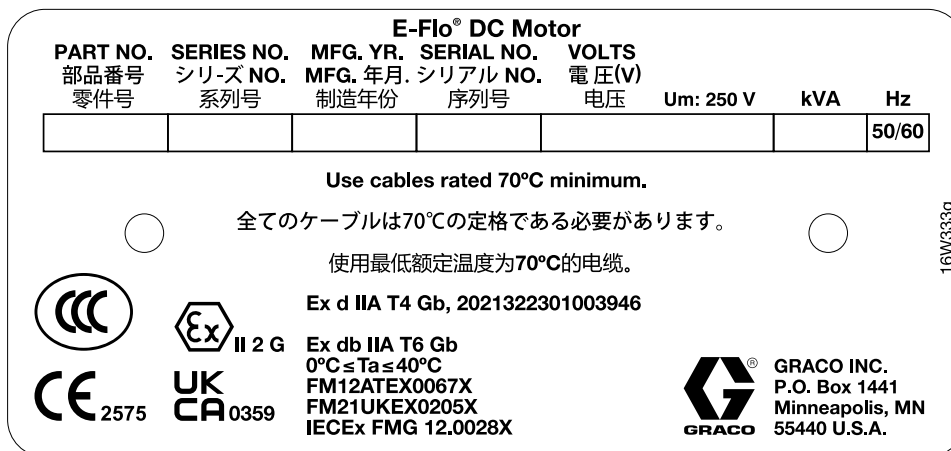
Figure 2 Basic-Motor mit regionsspezifischen Zulassungen Typenschild
