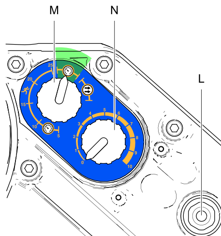
Figure 11 Druckmodus
