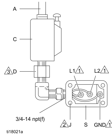
Figure 7 Anschließen der Stromkabel
