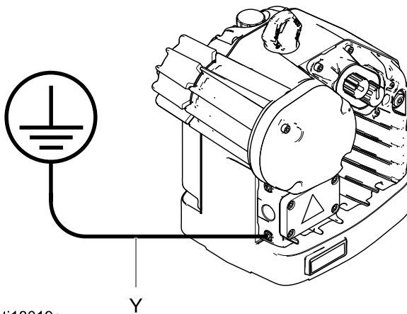
Figure 8 Erdungsleitung
