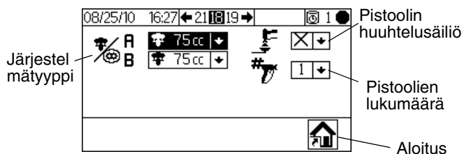
Kuva 36. Konfigurointi 1 (näyttö 18)
