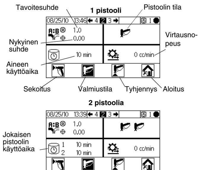
KUVA 26. Aja ruiskutuksen sekoitus (näyttö 2)
