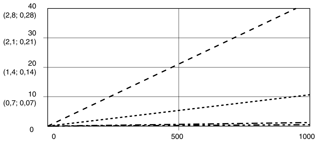
KUVA 59. Dynaaminen annostelu (30:1 suhde, 90 cP neste, 100 psi A-puolen paine)
