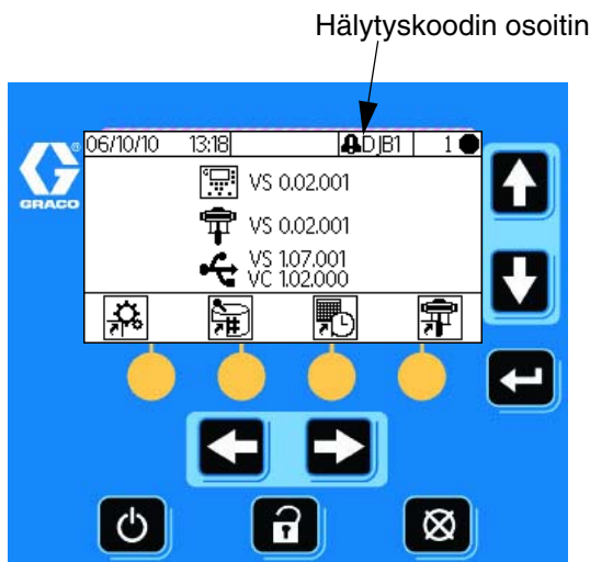
KUVA 53. Näyttöyksikön hälytyskoodit
