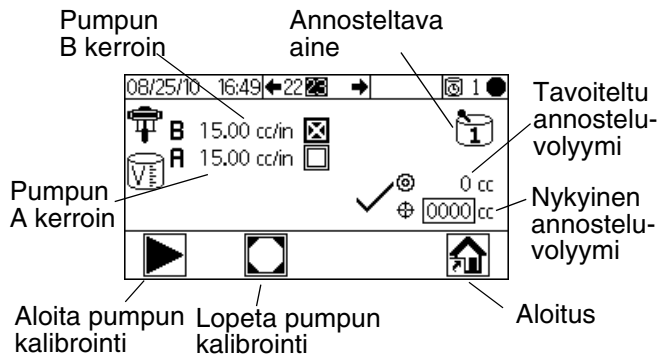
Kuva 44. Kalibrointi 2 (näyttö 23)
