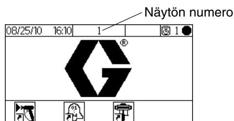
KUVA 27. Ajotilat koti (näyttö 1)
