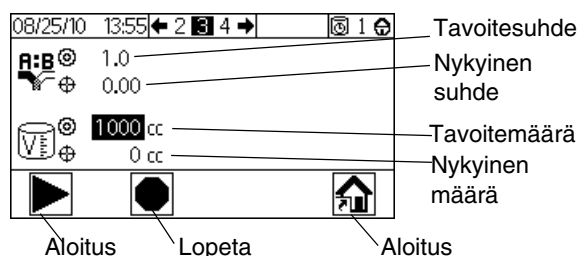
KUVA 28. Aja sekoituserä (näyttö 3)
