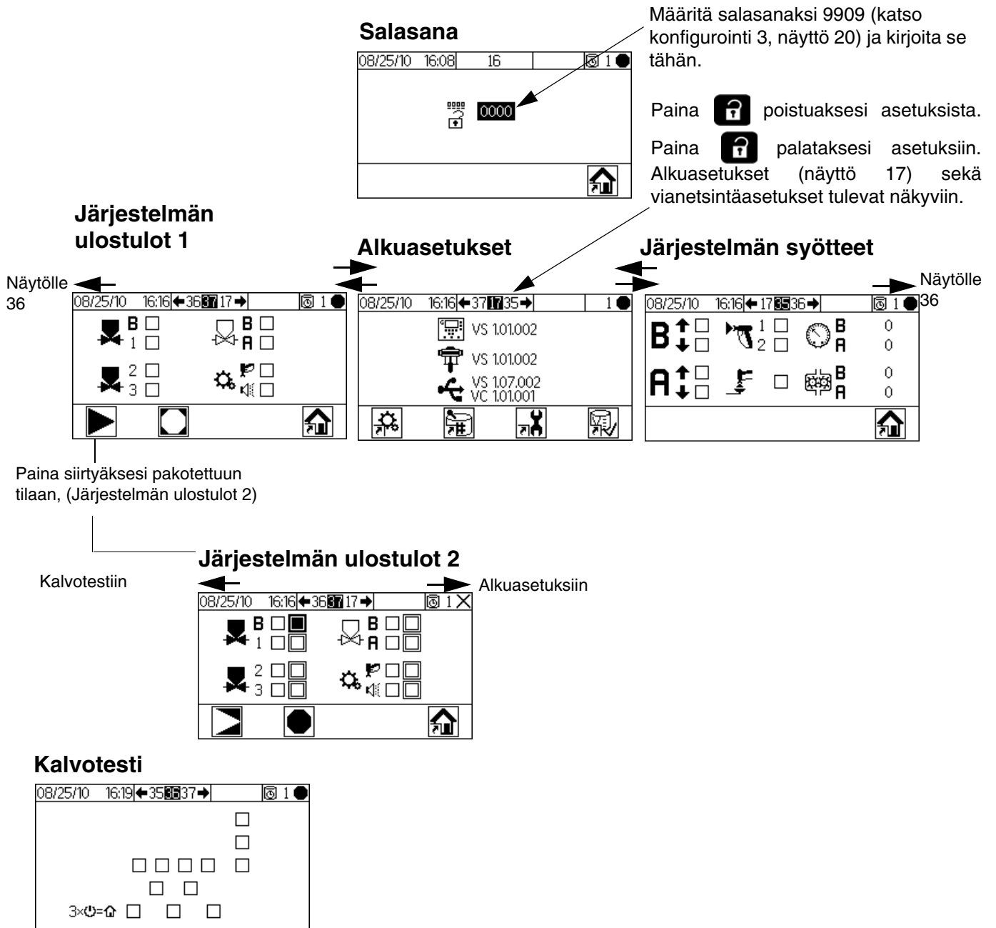
KUVA 14. Vianetsintänäkytön kartta
