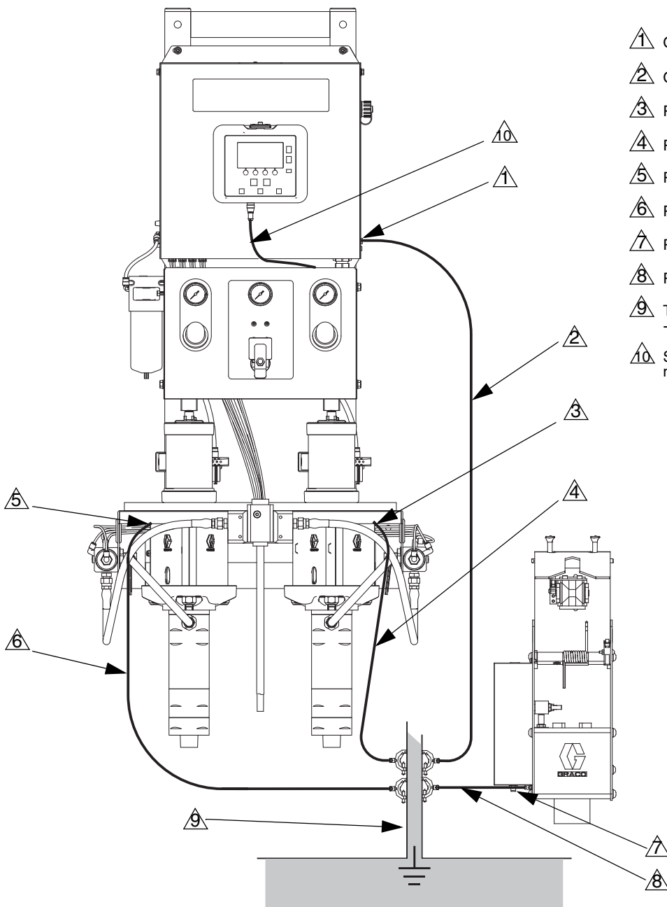
KUVA 9. Maadoitus
