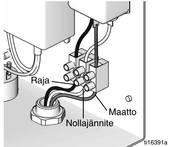
KUVA 6. Sähköohjauskeskuksen sähköliitäntä
