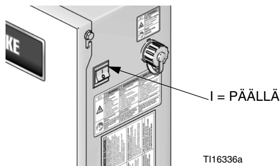
Kuva 15. Virtakytkin
