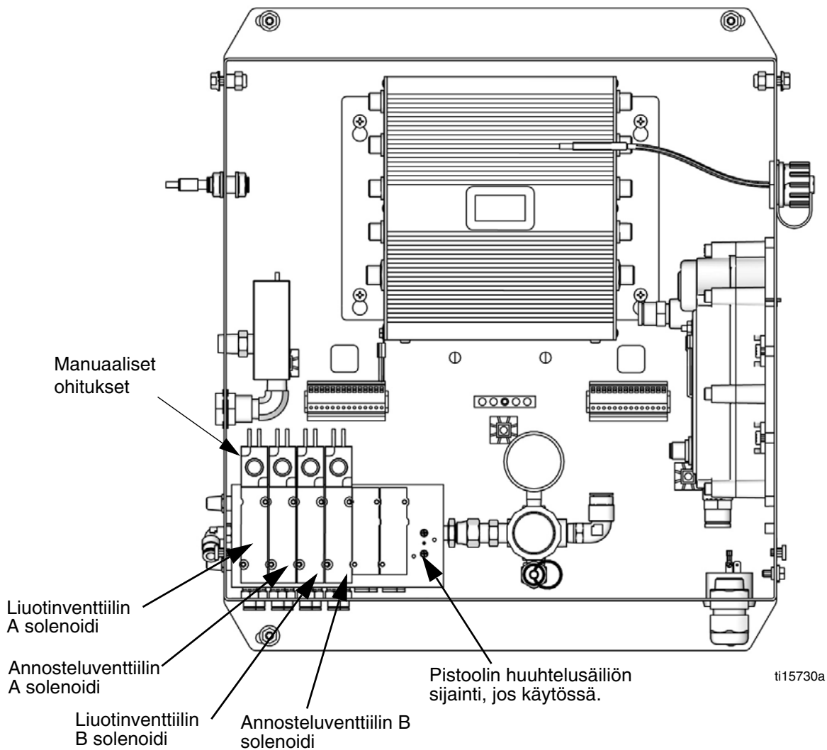
KUVA 19. Solenoidiventtiilit ohjausrasiassa
