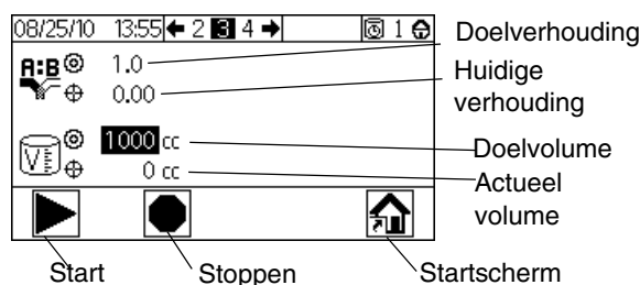
AFB. 28. Mengbatch uitvoeren (scherm 3)
