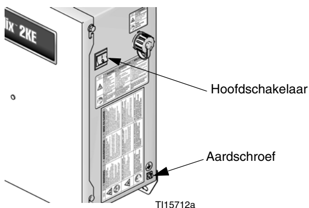
AFB. 8. Aardingschroef en voedingschakelaar
