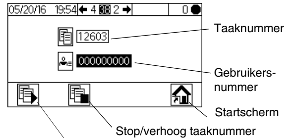
AFB. 31. Taaknummer uitvoeren (scherm 38)
