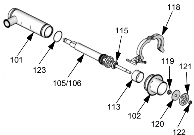
FIG. 2. Retiro de la varilla del pistón
