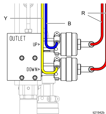
Figure 22 Schlauchanschlüsse am Auslassverteiler
