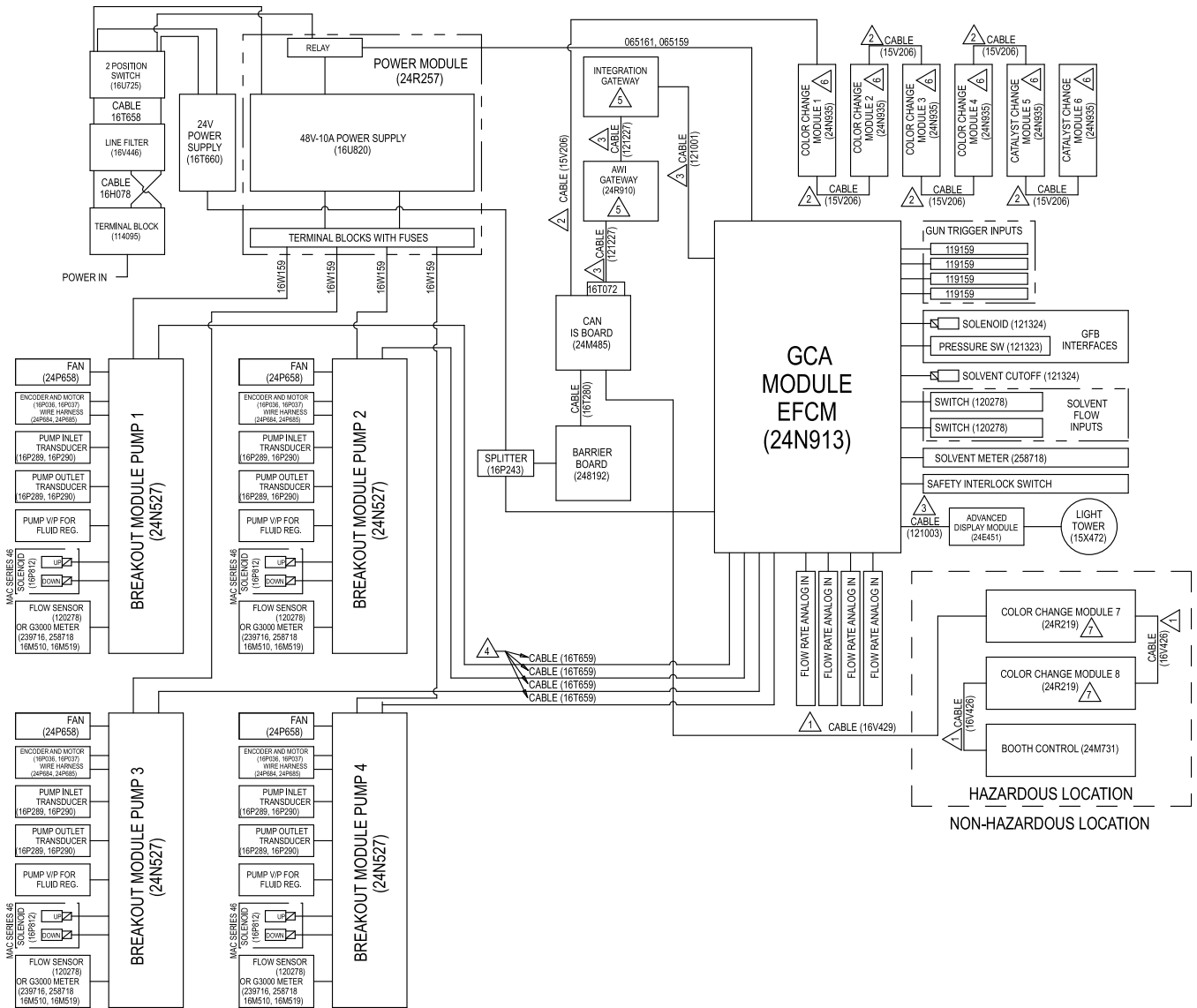
Figure 26 Schaltbild, Blatt 1
