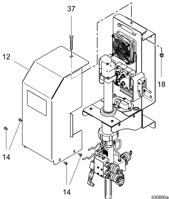
Figure 14 Abdeckung von Nachrücksatz installieren (Wandmontage)
