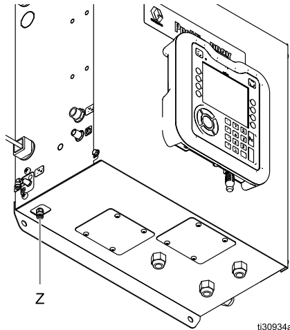
Figure 5 Luftanschluss für den ersten Nachrüstsatz des PD1K
