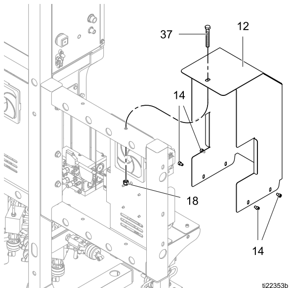
Figure 13 Abdeckung von Nachrücksatz installieren (Rahmen)
