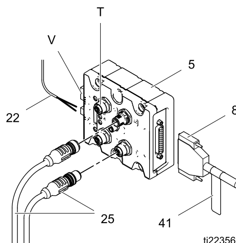
Figure 25 Anschlüsse des Pumpenregelmoduls
