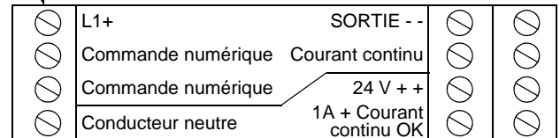
Détails du câblage d'alimentation électrique
