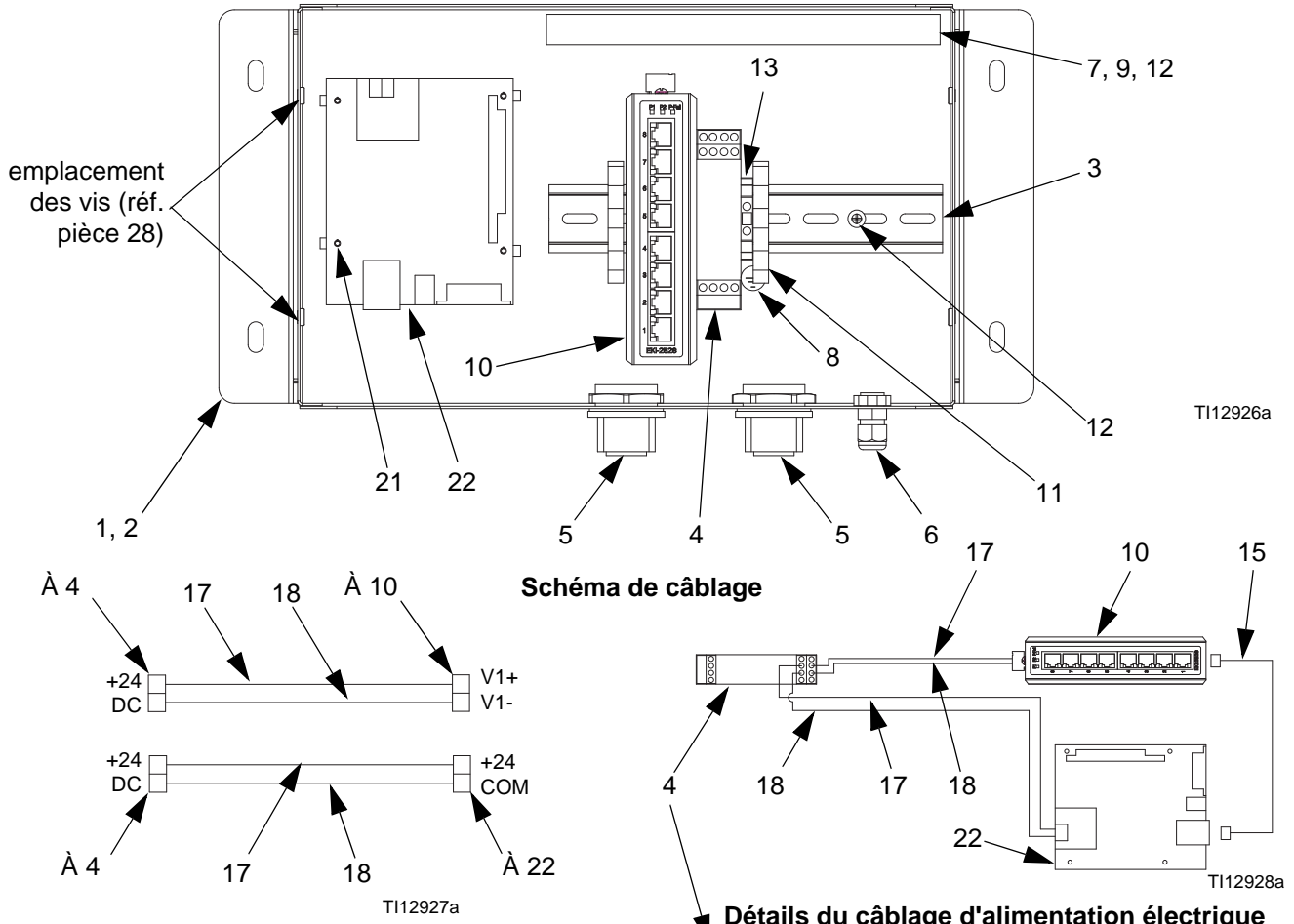
Détails du câblage d'alimentation électrique
